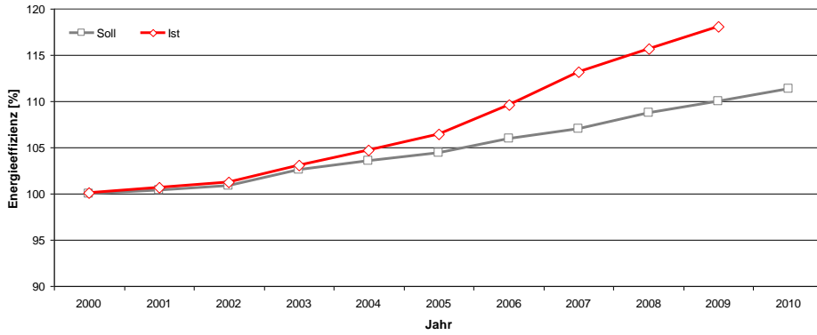
Energieeffizienz (HGT-normiert)
